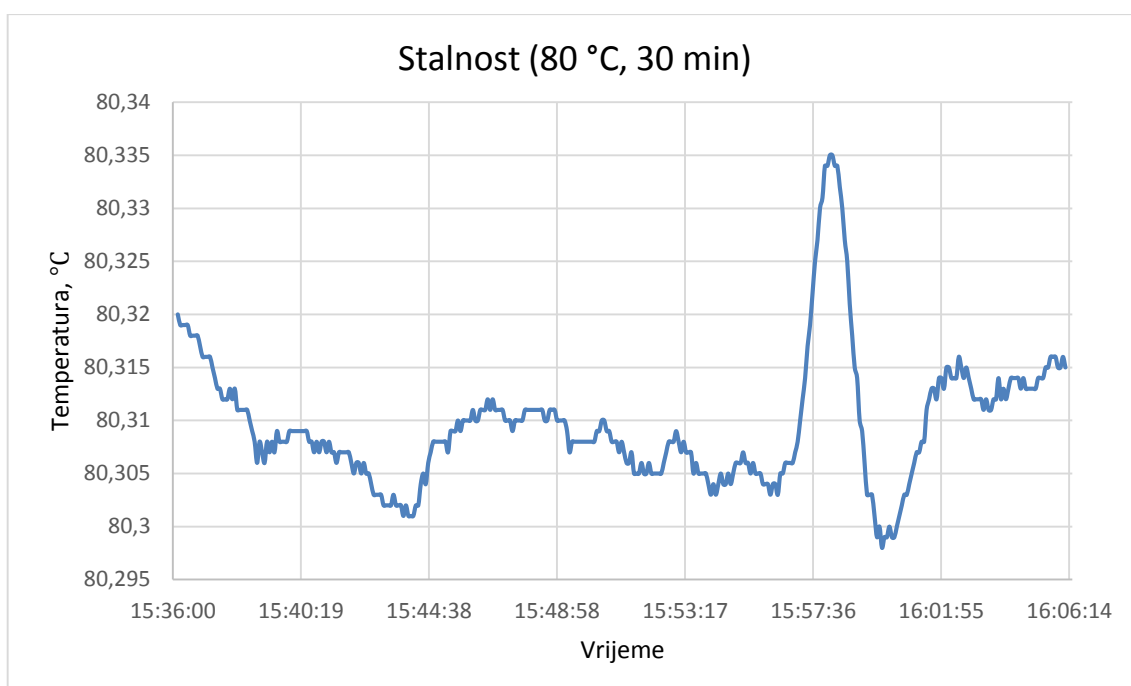
Slika 13. Dijagramski prikaz stalnosti temperature za 80 °C
