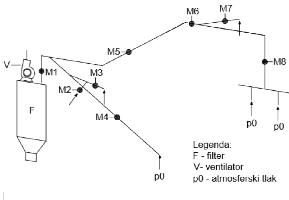
Slika 9. 2-D shema postrojenja sa označenim mjernim mjestima
