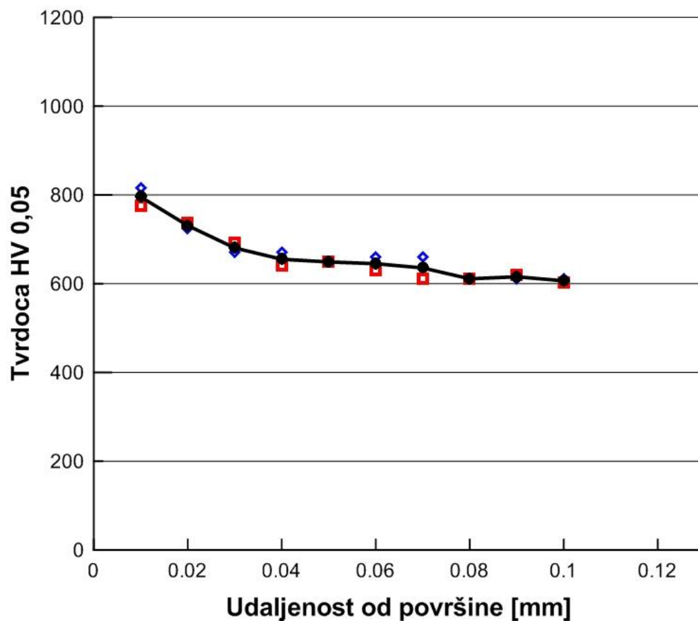
Slika 66. Raspored mikrotvrdoće po poprečnom presjeku uzorka B1 (nitirano)
