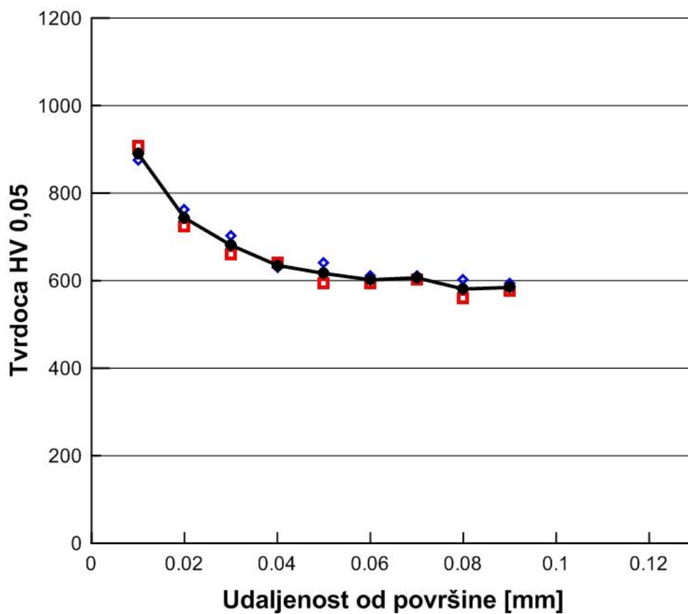
Slika 67. Raspored mikrotvrdoće po poprečnom presjeku uzorka B2 (nitirano + TiCN prevlaka)
