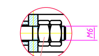
DETALJ H (M1:1)
