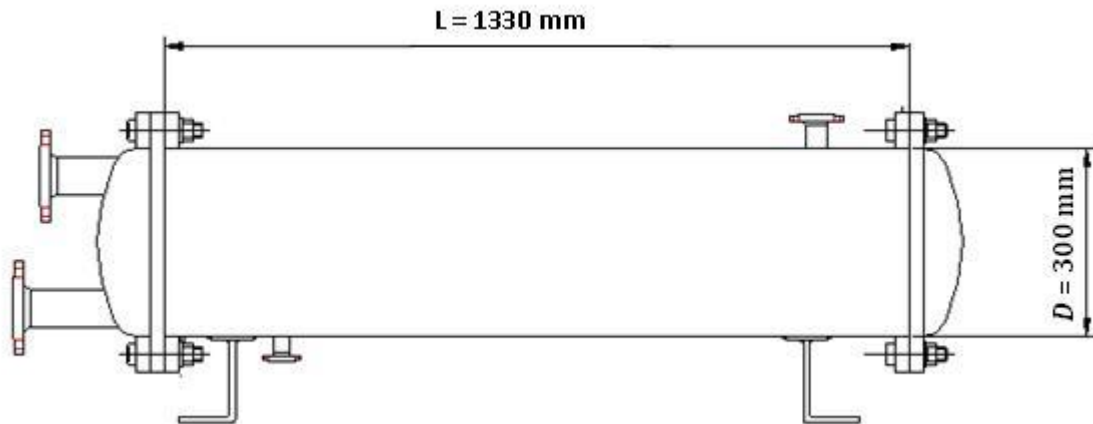
Slika 20. Dimenzije kondenzatora
