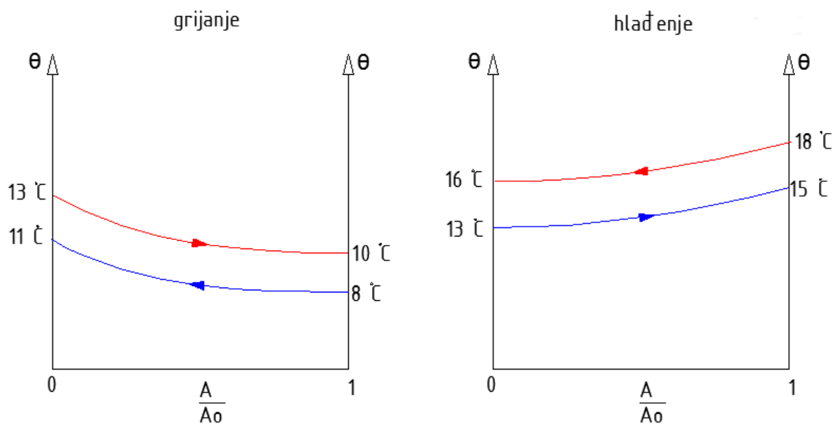
Slika 26. Dijagram međuzmjenjivača
