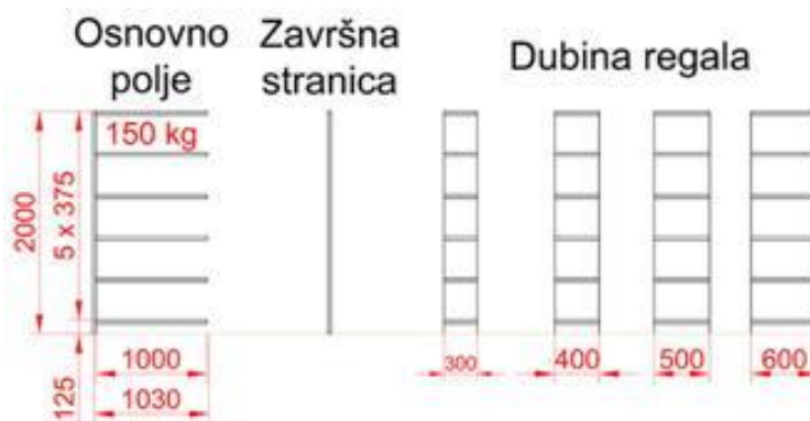
Slika 11. Lagani regali [5]
