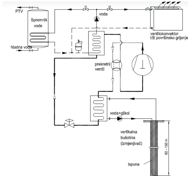
Slika 10. Dizalica topline s tlom kao toplinskim spremnikom-horizontalna izvedba [3]
