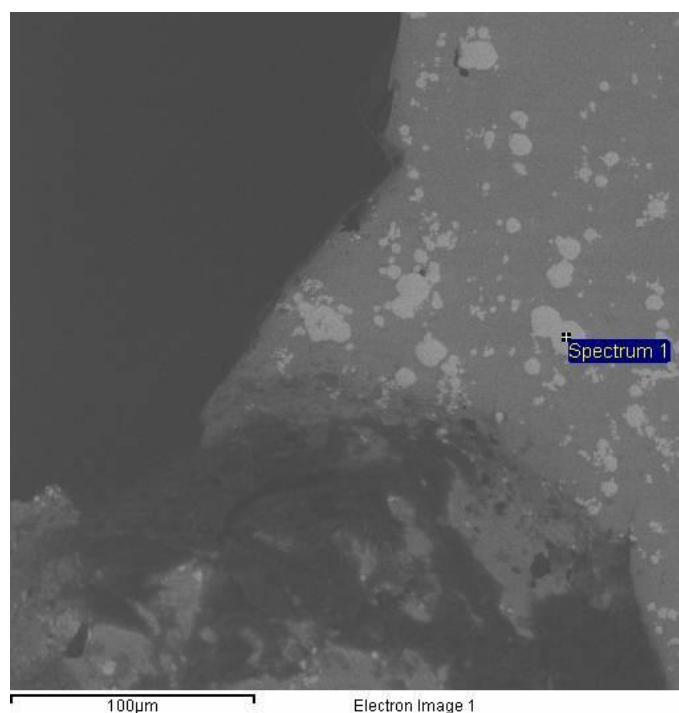
Slika 37. EDS analiza najzastupljenijeg elementa matrice, rezne pločice
