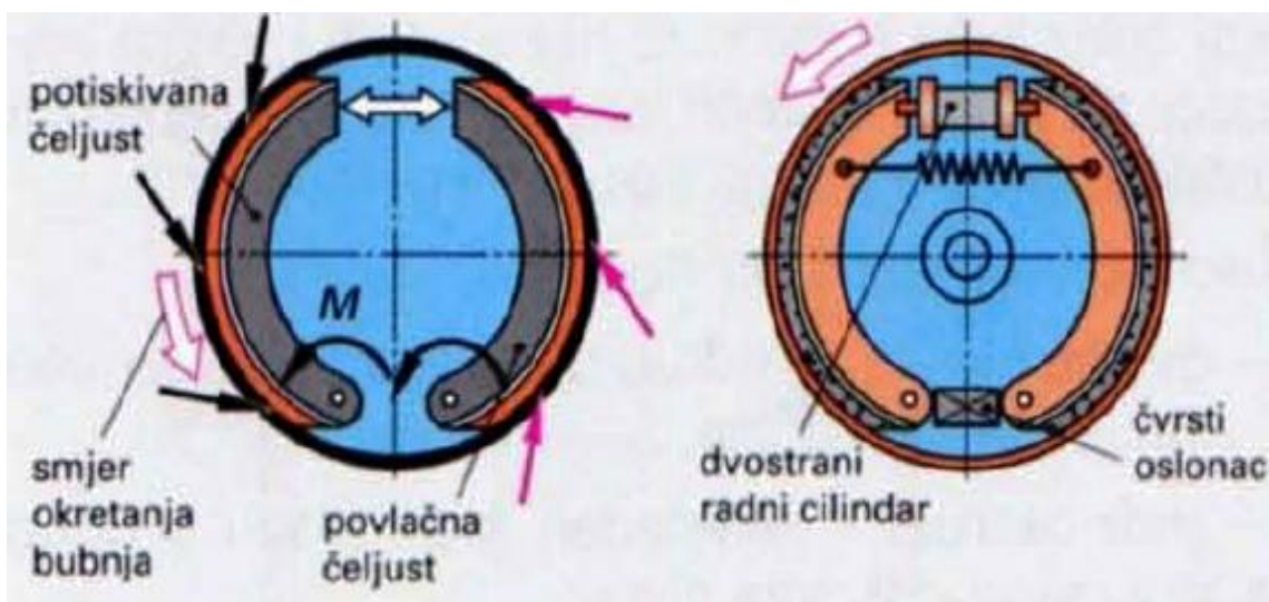
Slika 39. Simpleks kočni bubanj
