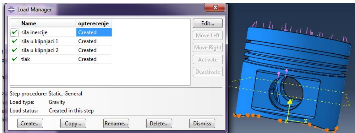
Slika 4.9. Opterećenja na klipju pri 360° KV.
