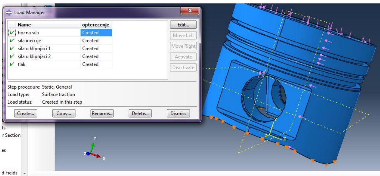
Slika 4.10. Opterećenja na klipju pri 372° KV.
