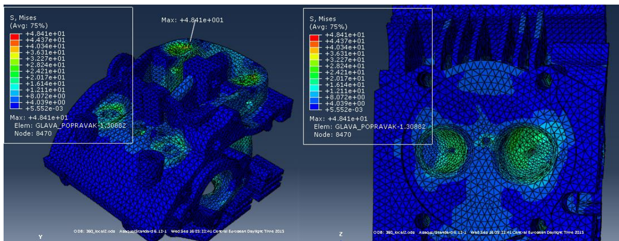
Slika 4.36. Ekvivalentna napreznja glave motora pri 360° KV.
