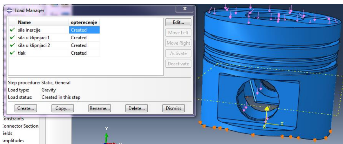
Slika 4.8. Opterećenja na klipu pri 0^\circ KV.
