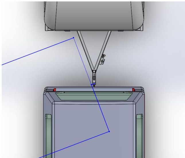
Slika 45. Provjera skretanja
