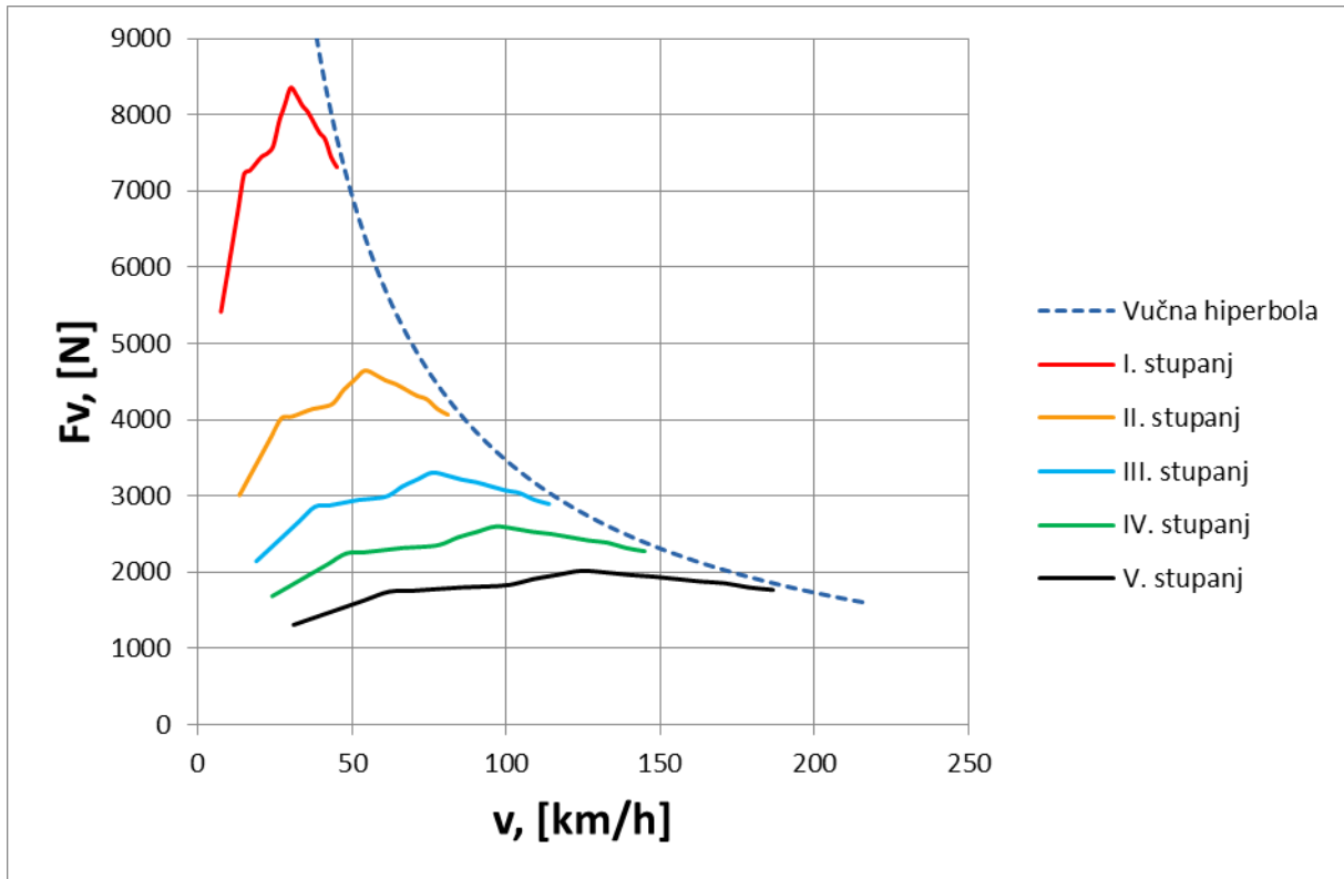
Slika 30. Vučni dijagram
