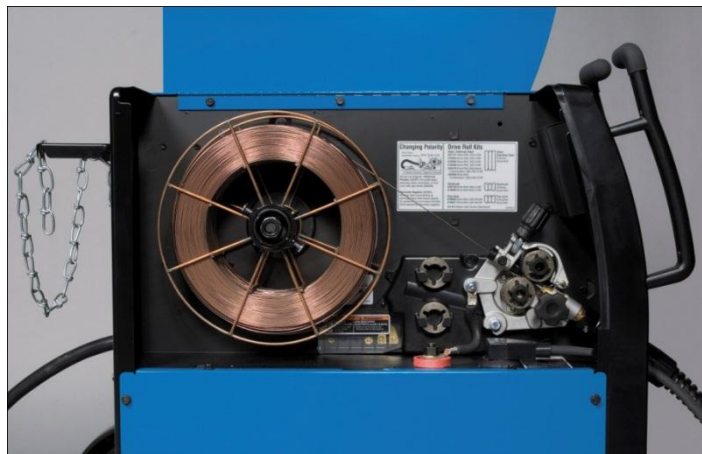
Slika 11. Unutrašnjost dodavača žice [10]
