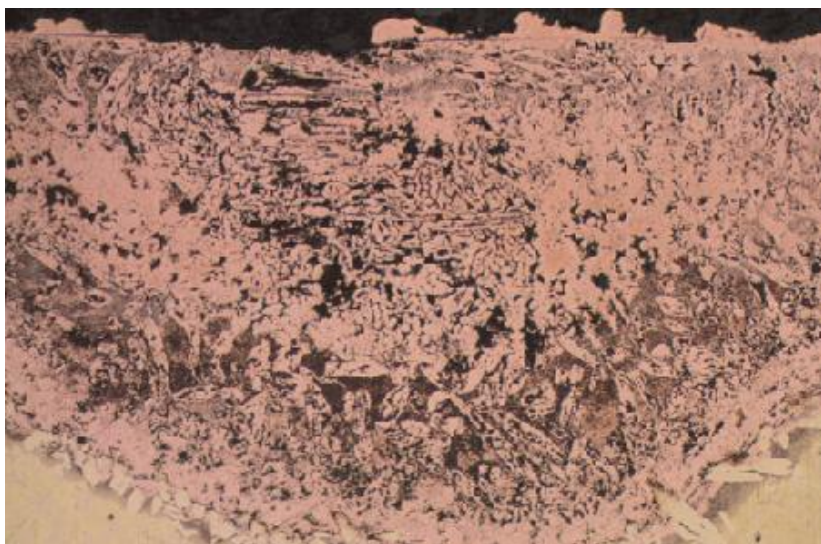
Slika 2.7. Decinkacija mjedi [15]
