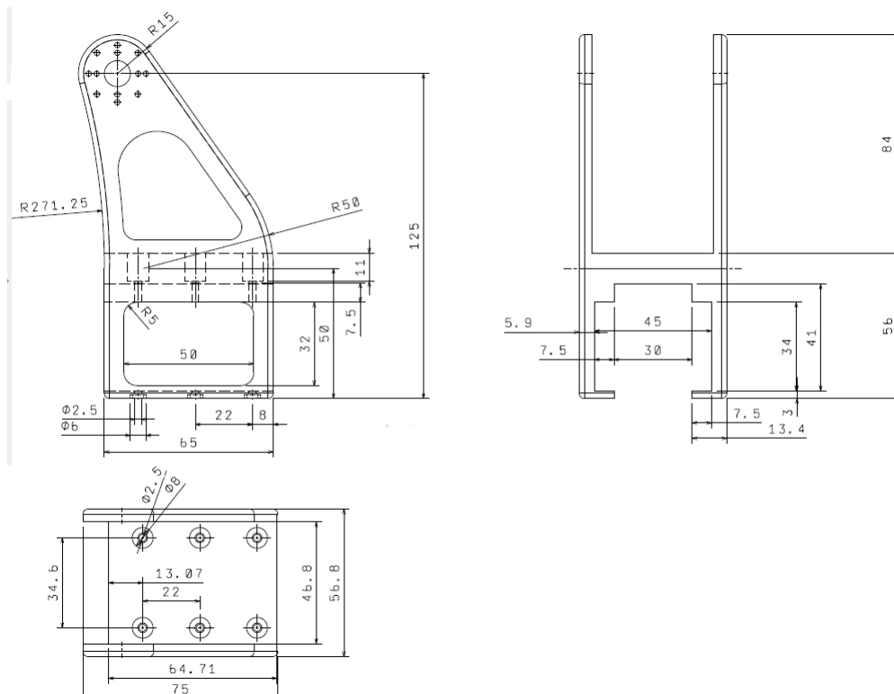
Slika 19: Dimenzije kralježnice
