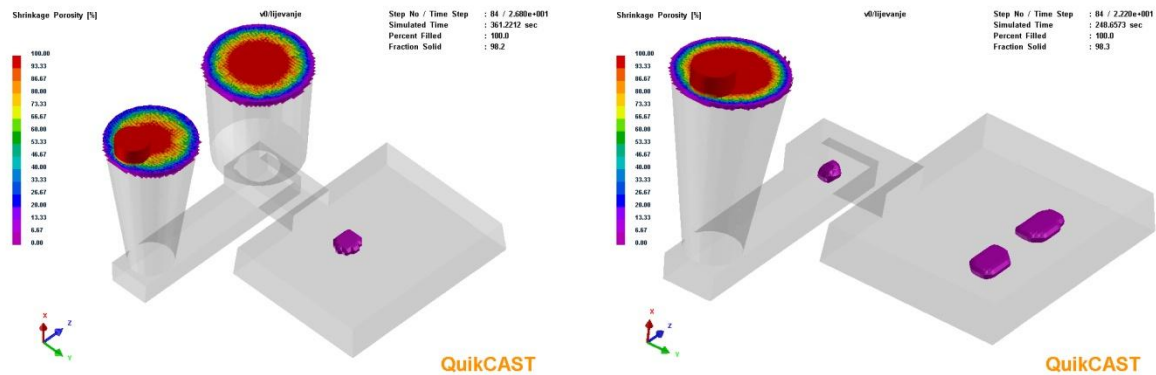
Slika 41: Poroznost u odljercima s horizontalnim uljevnim sustavom s jednim ušćem i toplim pojilom te bez nje
