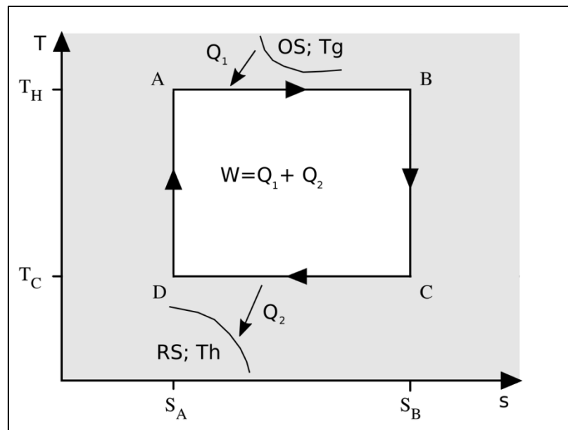
Slika 2. Carnot-ov proces
