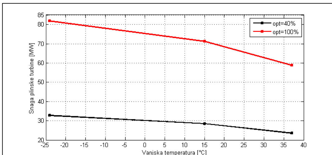
Slika 25. Proizvedena toplina bloka K iz kotla na opadnu toplinu za zagrijavanje topl vodne mrežne vode u ovisnosti o vanjskoj temperaturi i opterećenju
