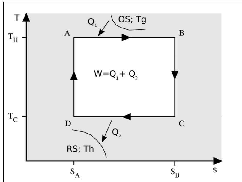
Slika 2. Carnot-ov proces
