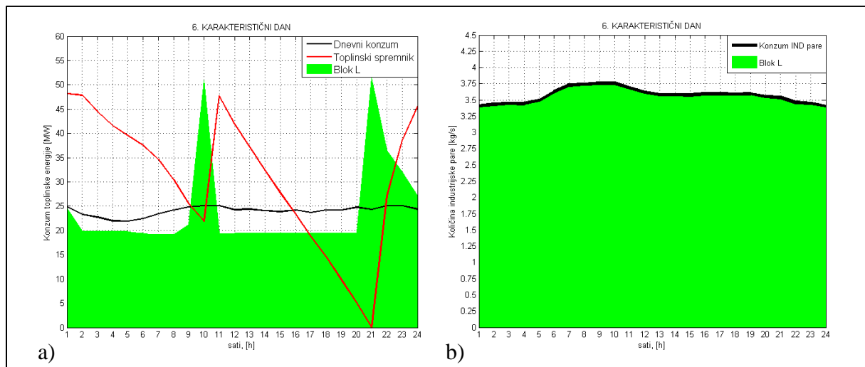
Slika 61. Udio pojedinih blokova u zadovoljavanju toplinskog konzuma (a) i konzuma industrijske pare (b) za šesti karakteristični dan
