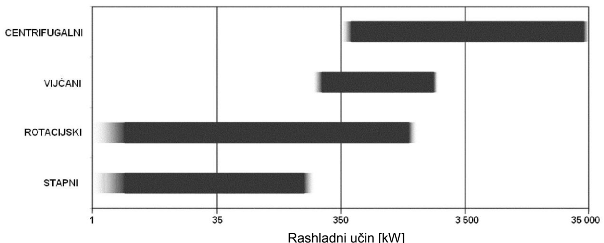
Slika 5.3. Tip kompresora u zavisnosti o rashladnom učinu [21]
