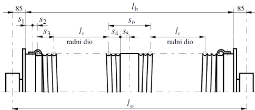
Slika 5.5. Dimenzije bubnja [1]
