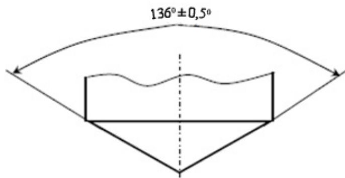
Slika 2.7 Dozvoljena odstupanja kuta nasuprotno ležećih stranica piramide [16]
