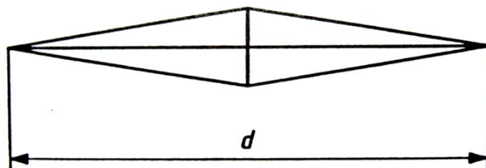
Slika 1.7 Izgled otiska indentora kod Knoopove metode [10]
