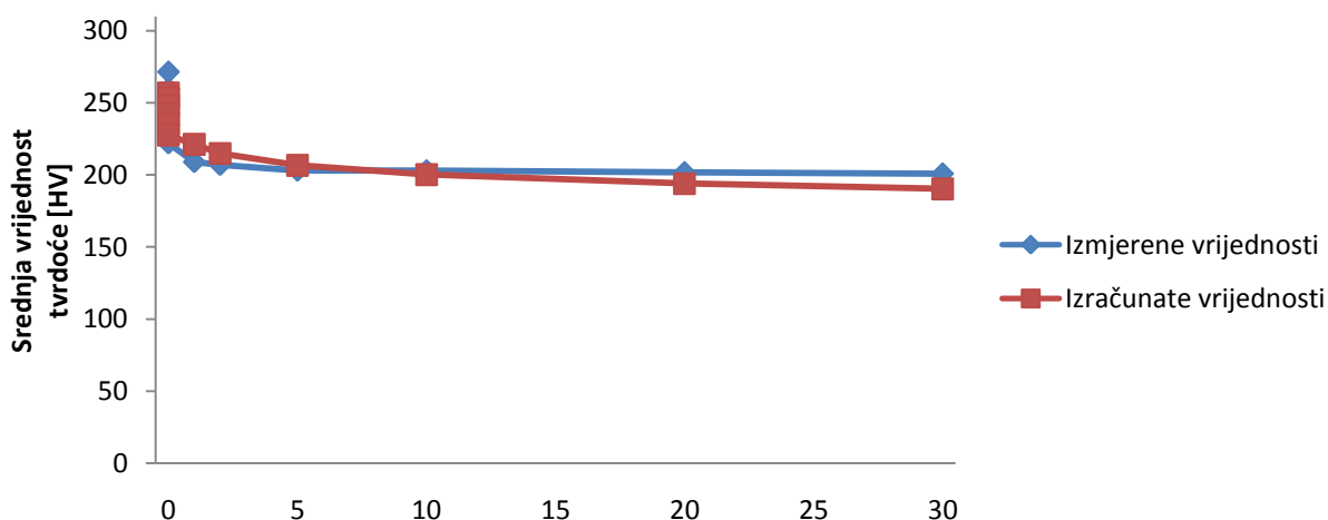
Slika 5.8 Razlika između izmjerenih i izračunatih vrijednosti tvrdoća
