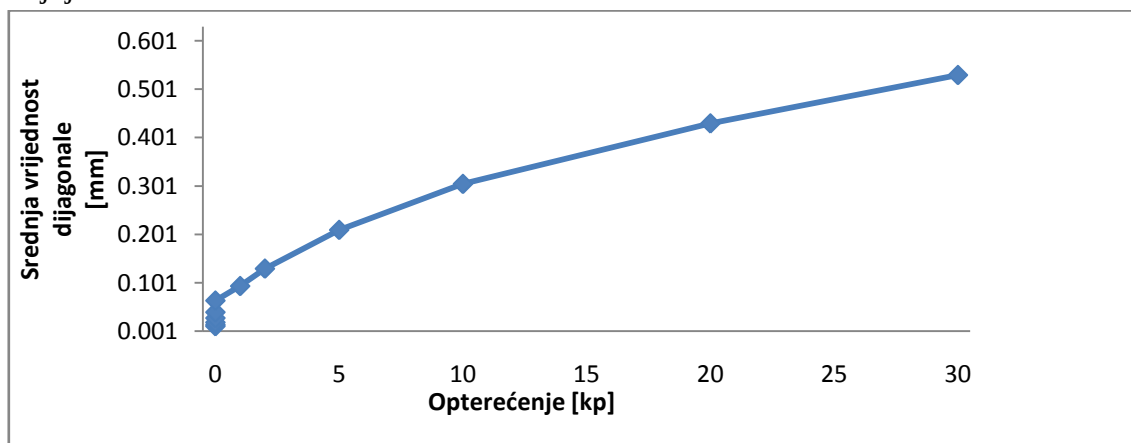
Slika 5.6 Promjena duljine dijagonale sa opterećenjem
