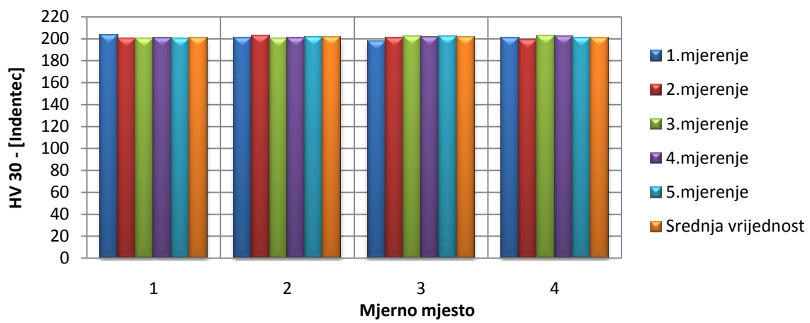
Slika 5.0 Prikaz rezultata mjerenja tvrdoće na tvrdomjeru 2 metodom HV30
