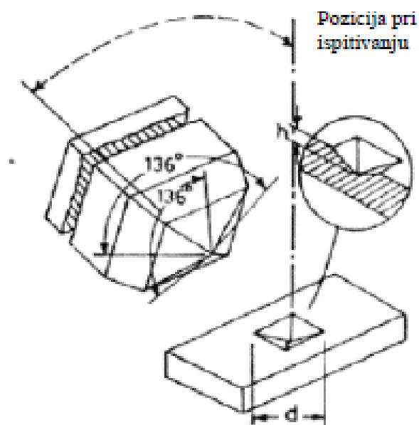
Slika 1.8 Dijamantna piramida kao indenter za Vickersovu metodu [13]
