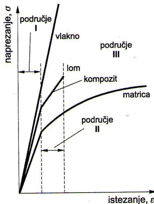
Slika 3. Dijagram "naprezanje-istezanje" vlaknima ojačanog kompozita [2]
