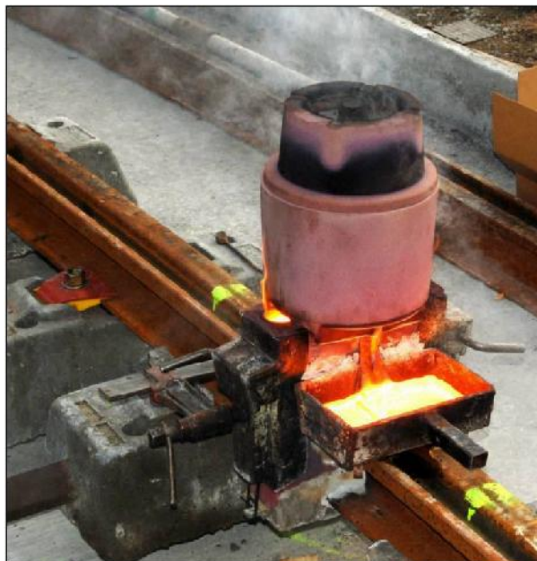
Slika 3.5. Zavarivanje tra nica aluminotermijskim postupkom [9]
