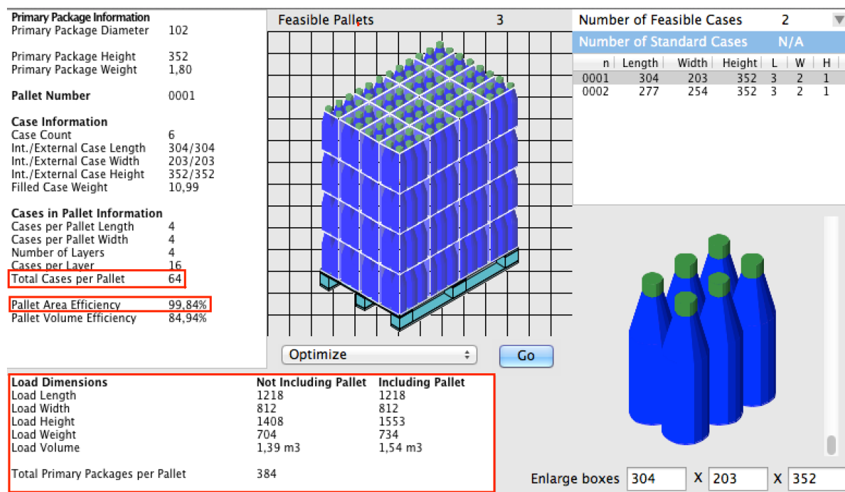
Slika 33. Raspored boca od 1,8 l na Euro paleti [14]
