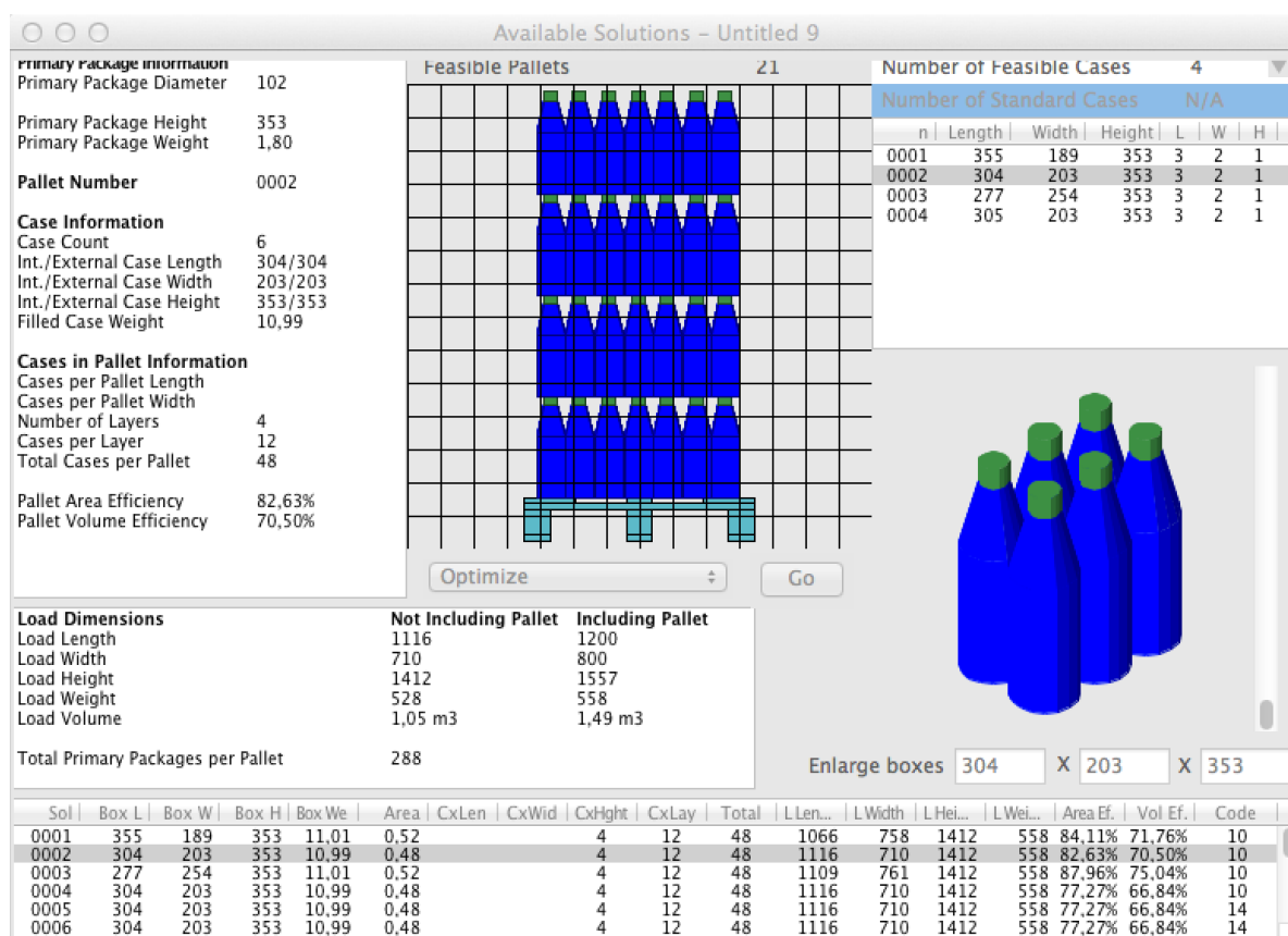
Slika 25. Primjer optimalnog slaganja boca na paletu korištenjem Quick Pallet Maker alata [14]
