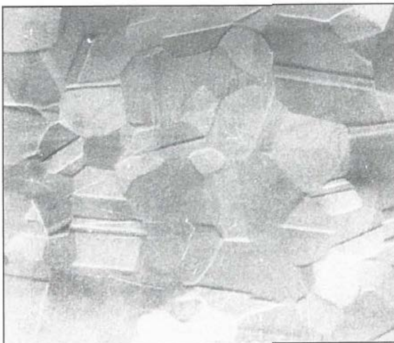
Slika 22. Mikrostruktura elektropolirane površine nehrđajućeg čelika [3]
