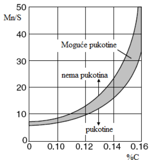
Slika 25. Odnos Mn/S u zavisnosti o %C na pojavu toplih pukotina [14]
