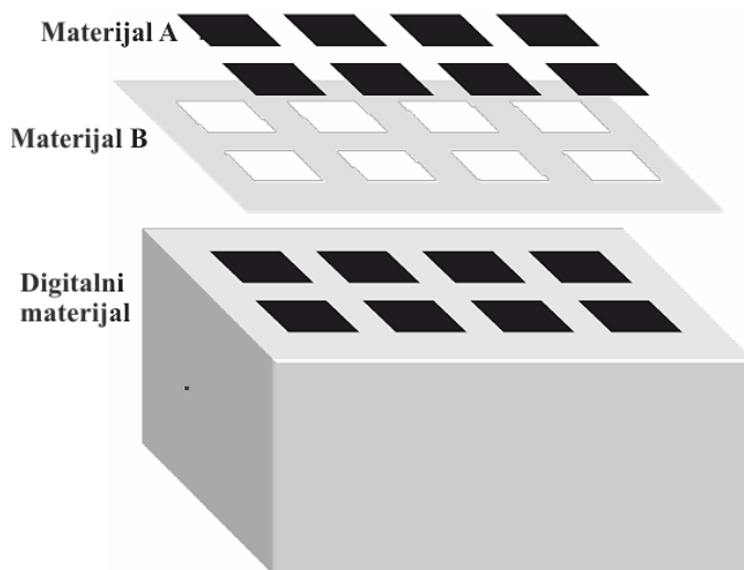
Slika 3.4. Digitalni materijal [17]
