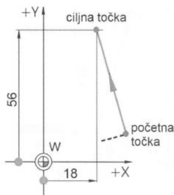
Slika 15. Apsolutni koordinatni sustav [2]
