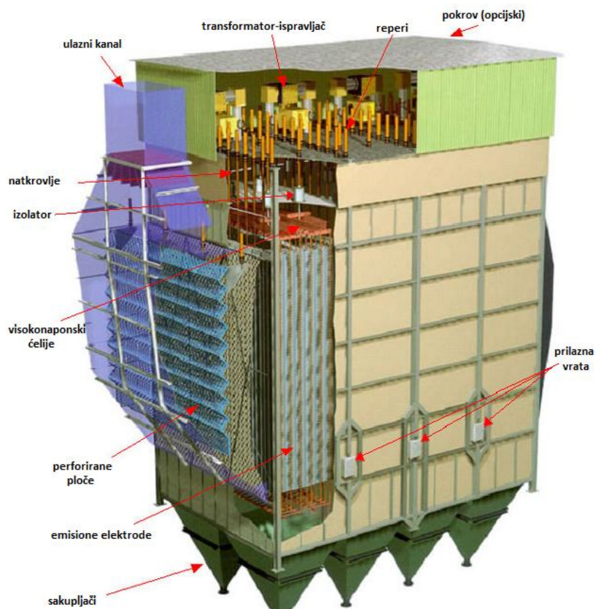
Slika 33. Elektro-precipitacijski filter [28]
