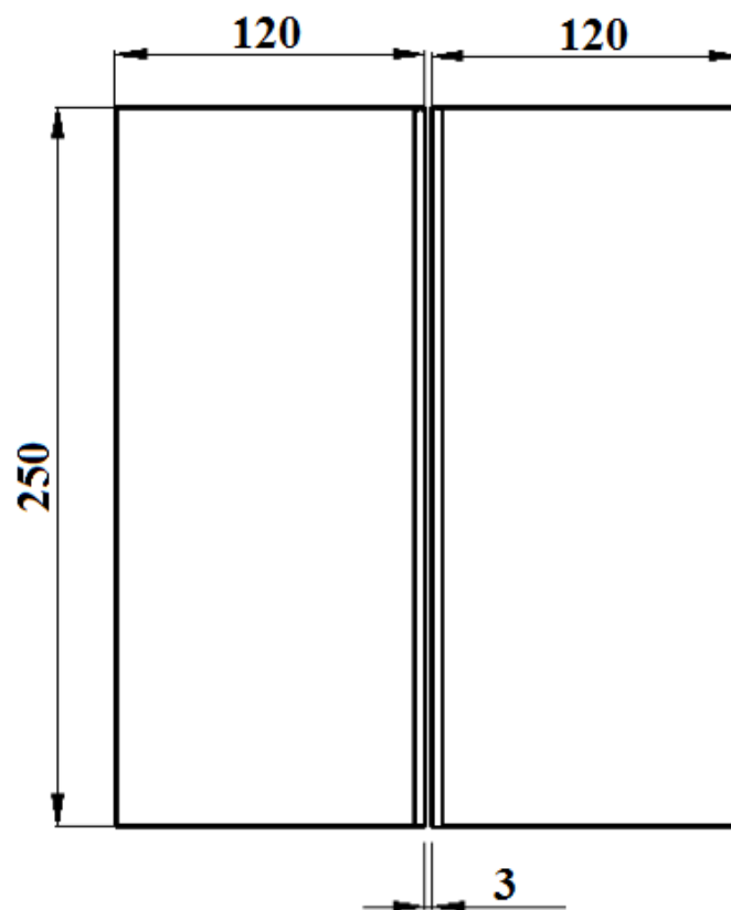
Slika 19 Dimenzije ploča
