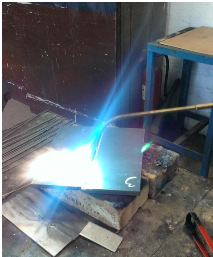
Slika 20 Predgrijavanje plinskim plamenom
