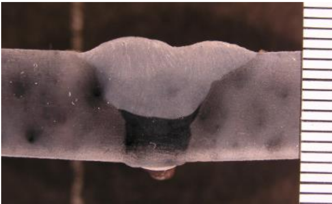
Slika 32 Makroizbrusak uzorka 2
