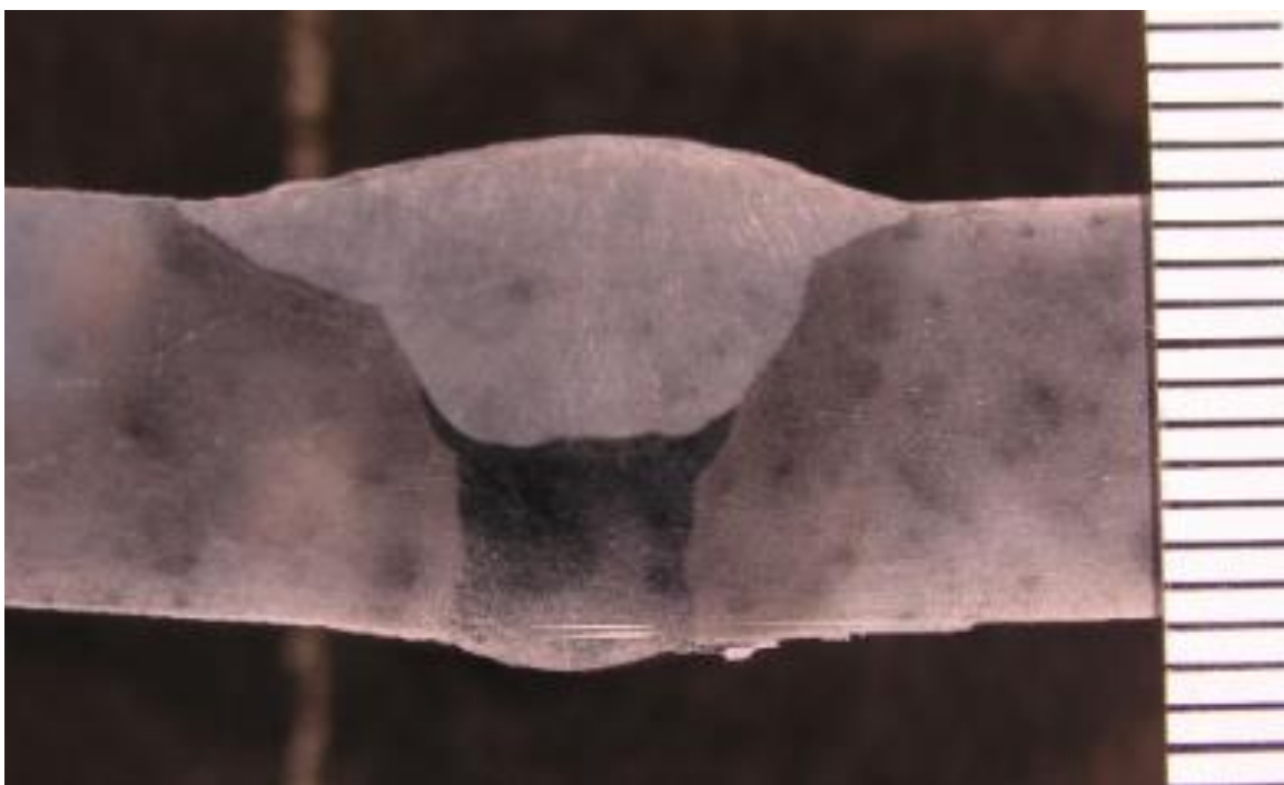
Slika 33 Makroizbrusak uzorka 3
