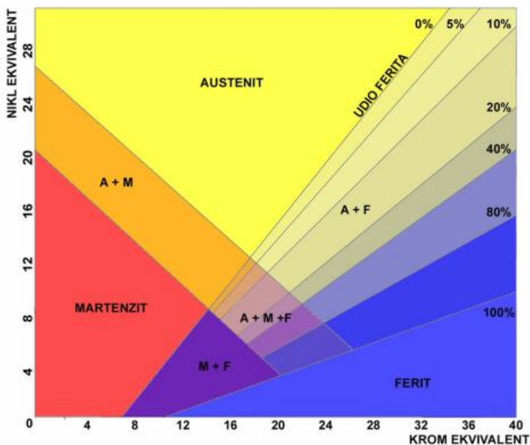
Slika 3 Schaefflerov dijagram [3]
