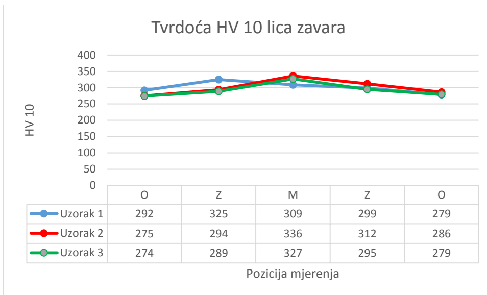
Slika 41 Grafički prikaz vrijednosti tvrdoća lica zavara
