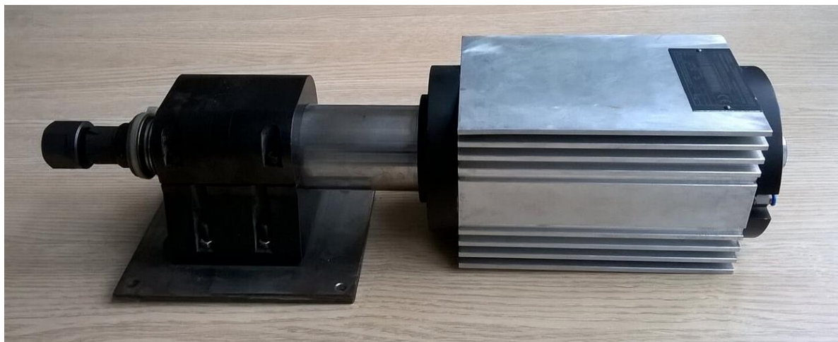
Slika 31. Fotografija motorvretena
