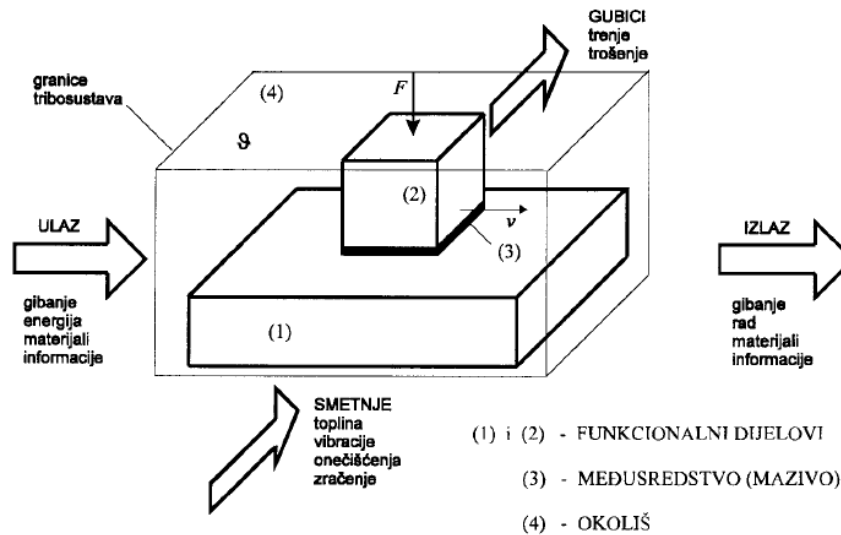
Slika 88. Tribološki sustav[30]
