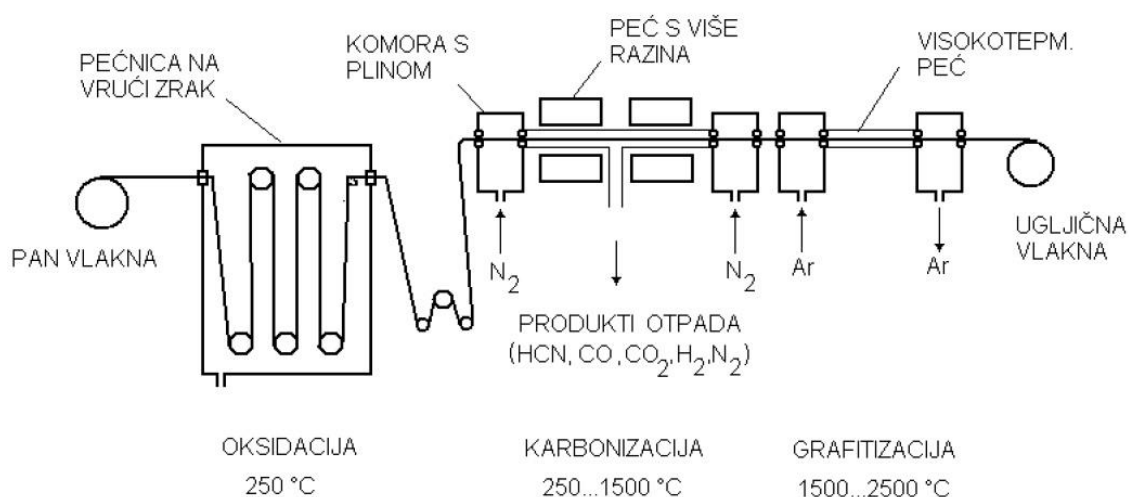
Slika 8 Postupak proizvodnje ugljičnih vlakana [7]
