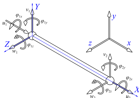
Slika 3.1. Osnovni prostorni gredni element
