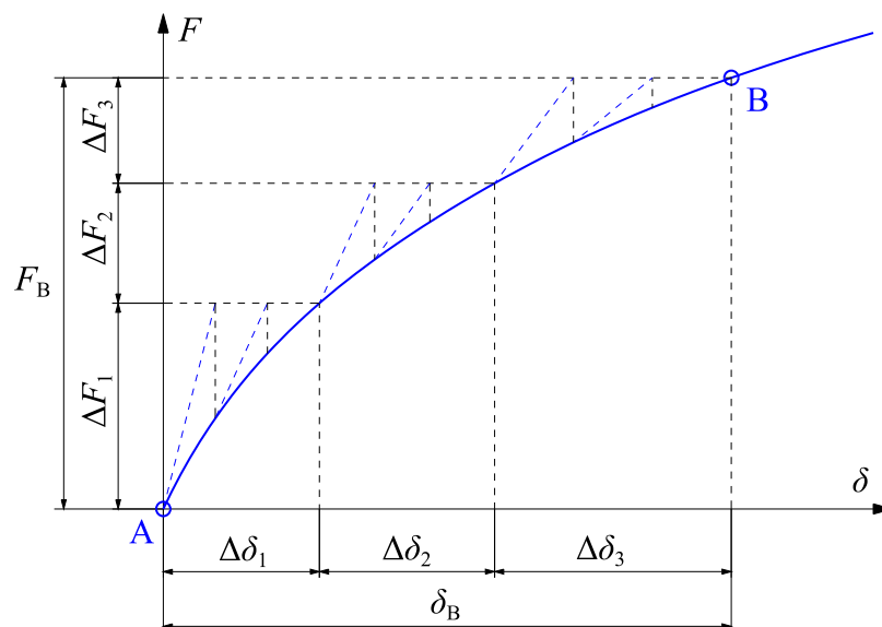
Slika 4.4. Kombinacija Newton-Raphson i inkrementalne metode
