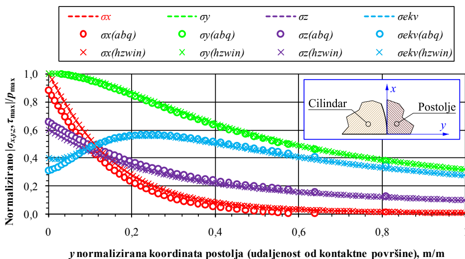
Slika 5.12. Usporedba normaliziranih rezultata napreznja: analitički model, HertzWin i Abaqus
