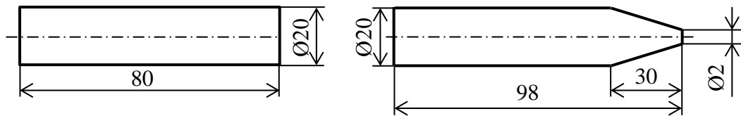
Slika 10. Geometrije projektila [4]
