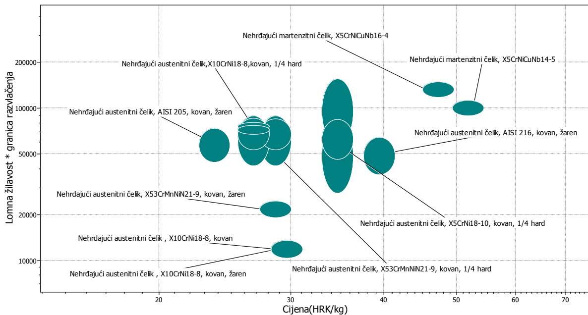
Slika 29. Dijagram cijena – lomna žilavost * granica razvlačenja [10]
