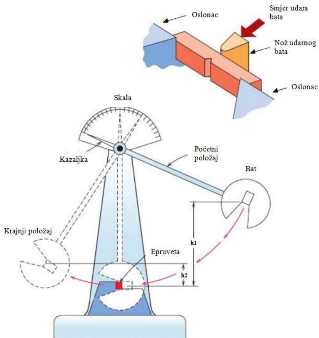
Slika 8. Charpy-ev bat [14]
