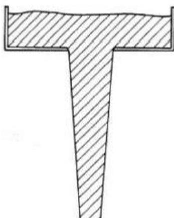
Slika 14. Pravilno konstruiran spust [11]
