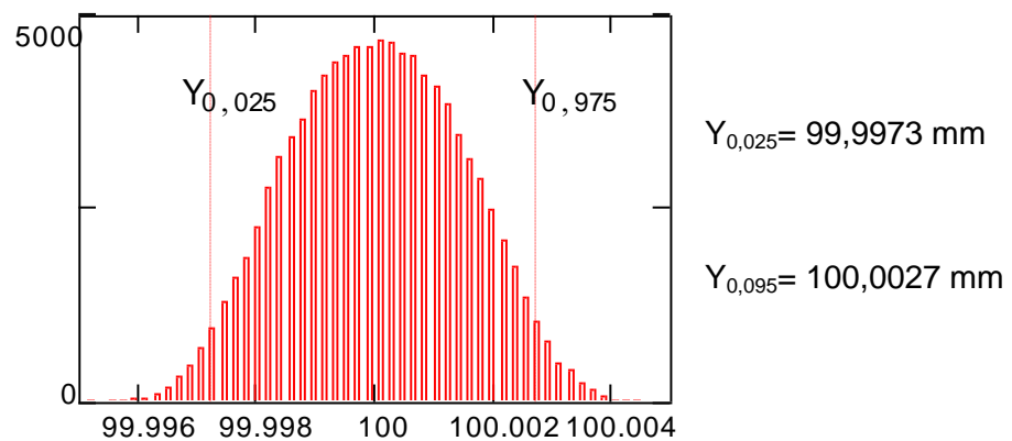
Slika 51. Funkcija gustoće vjerojatnosti g(L_x) za analognu uru rezolucije 0,01 mm i mjernog područja 100 mm [8]
