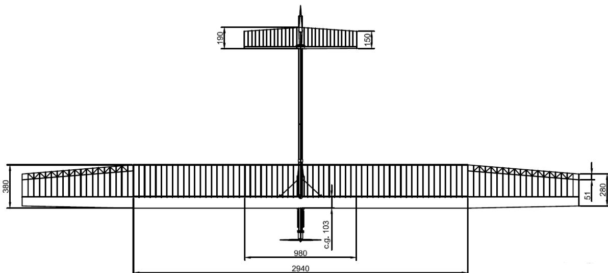
Slika 2.2 Tlocrt letjelice
