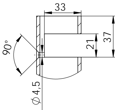
Detalj B M 1 : 2
