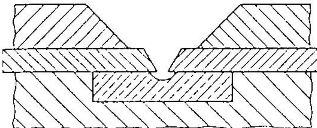
Slika 9. Bakrena pločica - akumulirani zaštitni plin [1]
