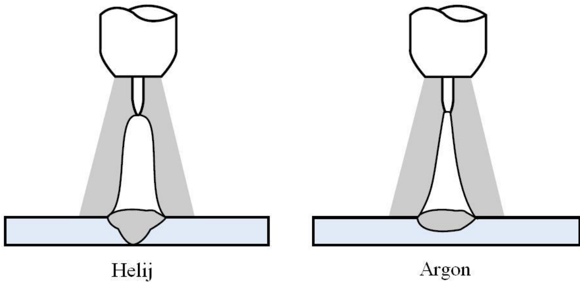
Slika 7. Usporedba zavarivanja s helijem i argonom [6]
