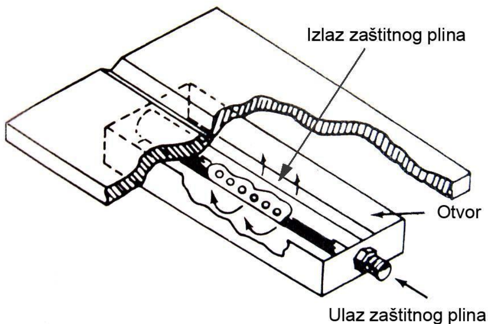
Slika 8. Zaštita korijena zavara u obliku kućišta [3]
