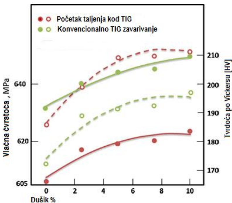
Slika 11. Utjecaj dodavanja dušika argonu na mehanička svojstva zavara [9]
