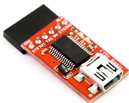
Slika 28. FTDI adapter [9]
