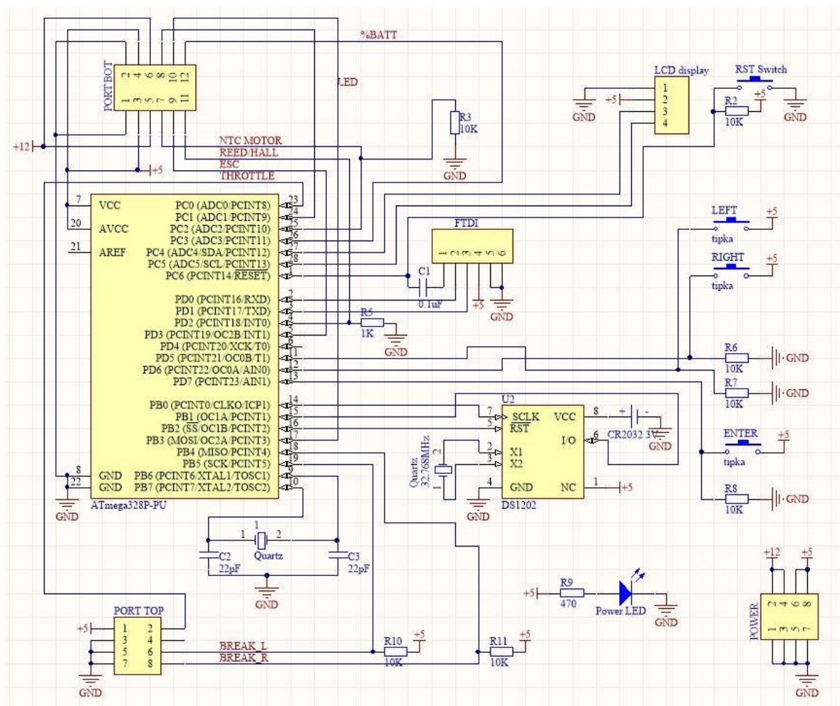
Slika 27. Shema donje pločice
