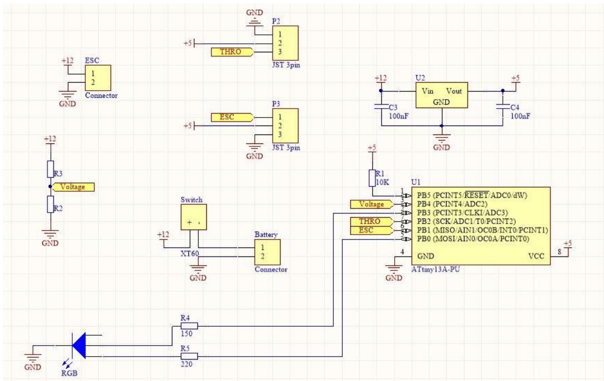
Slika 55. Električna shema pločice
