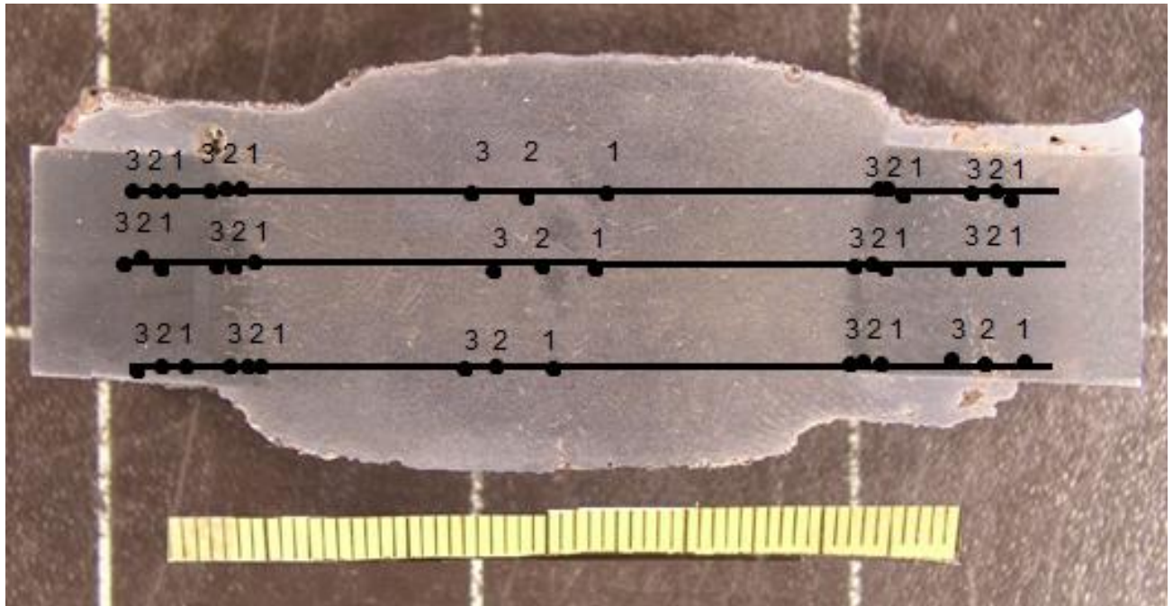
Slika 47 Makroizbrusak glave tračnice s lokacijama mjerenja
