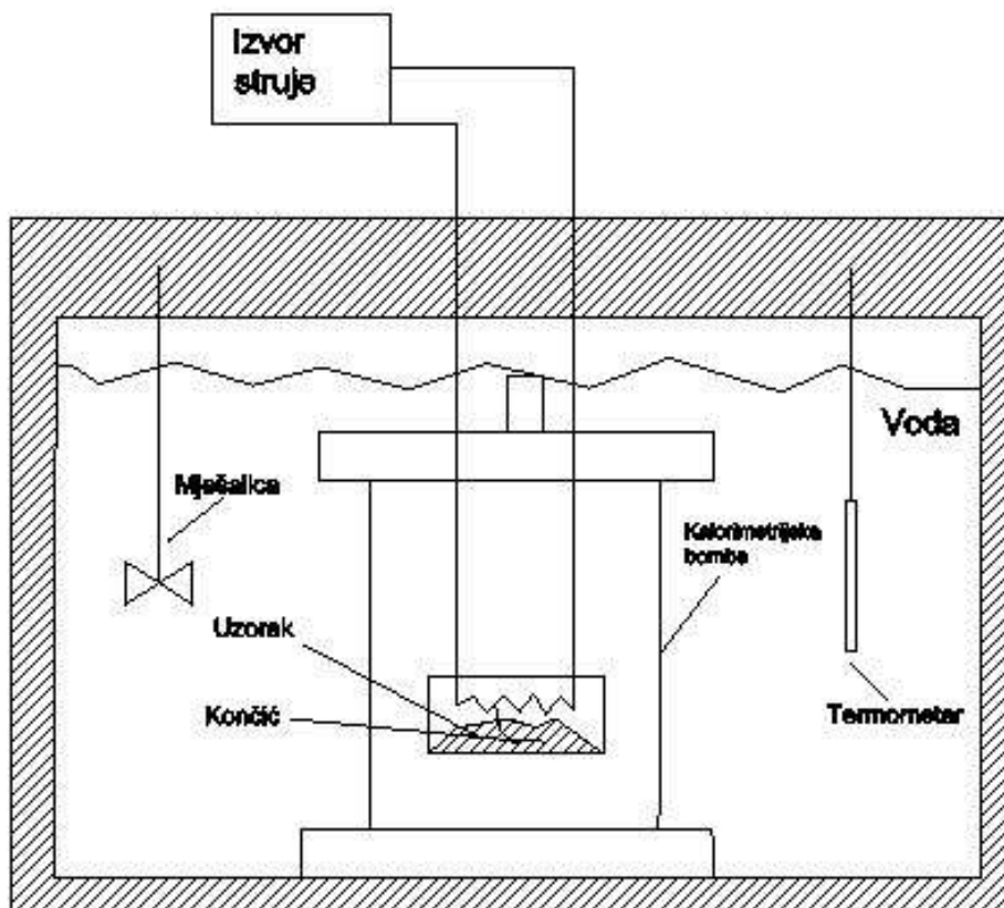
Slika 2.1. Shema adijabatskog kalorimetra
