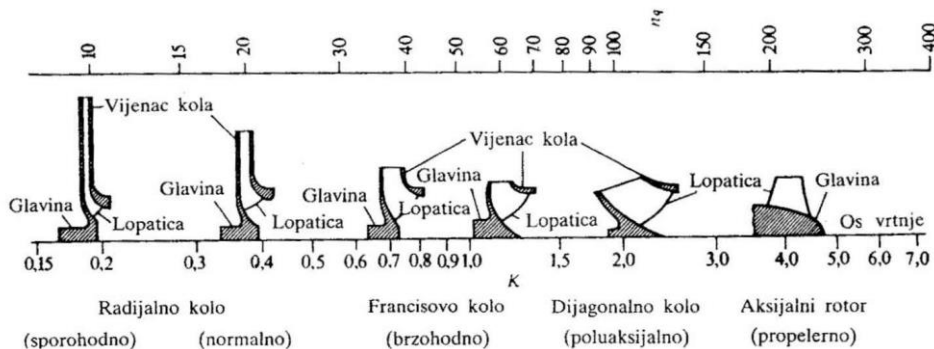
Slika 1.5 Ovisnost oblika rotora pumpe o brzohodnosti n_s
