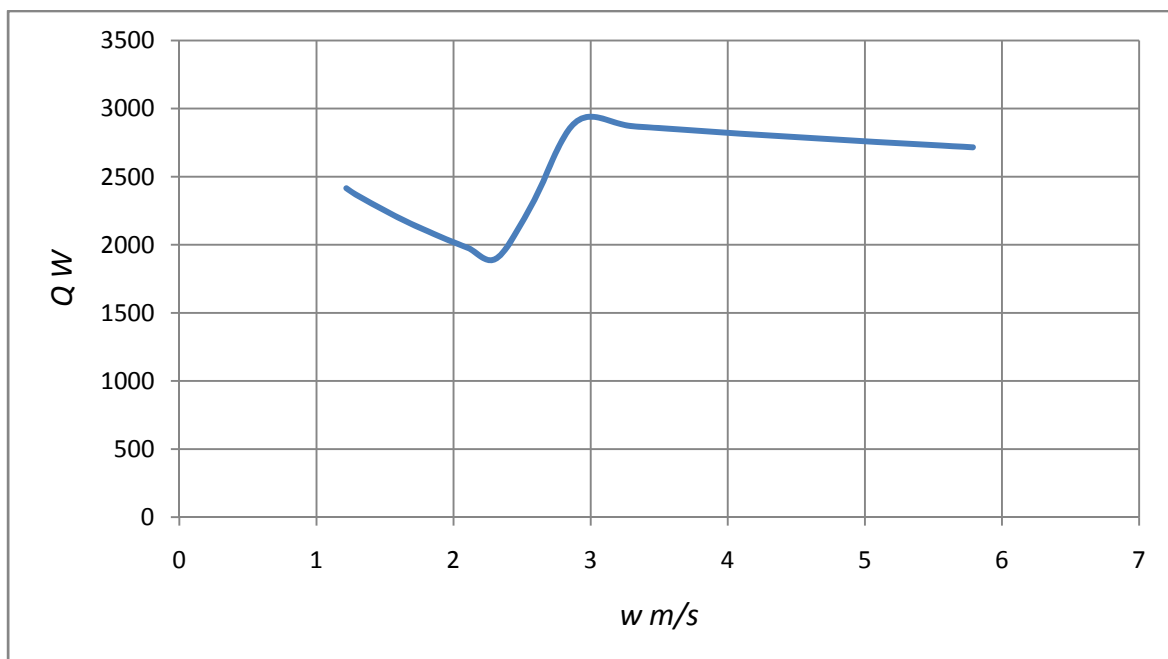
Slika 20. Ovisnost toplinskog toka Q o brzini strujanja uz protoke zraka q_v=500 \text{ m}^3/\text{h} i pri vanjskoj temperaturi \vartheta_1'=-15^\circ\text{C}
