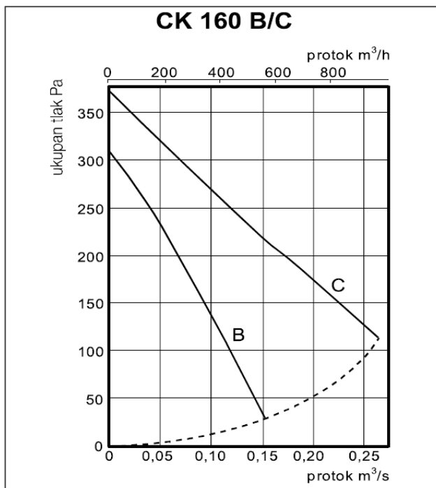
Slika 41. Karakteristika odabranog ventilatora
