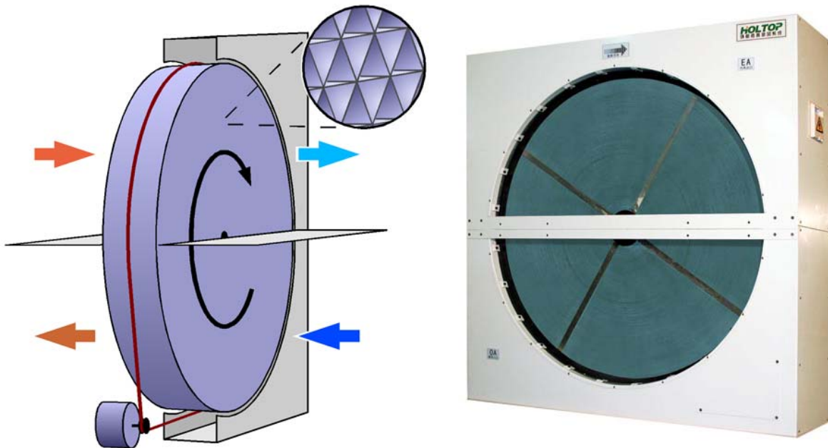
Slika 2. Rotirajući regeneratori
