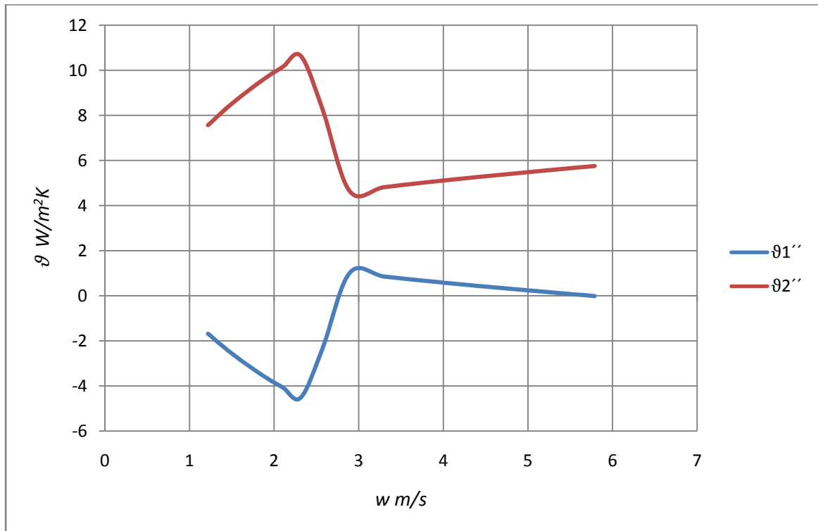
Slika 19. Ovisnost koeficijenta prijelaza topline o brzini strujanja pri protocima zraka q_v=500 \text{ m}^3/\text{h} i pri vanjskoj temperaturi \vartheta_1'=-15^\circ\text{C}
