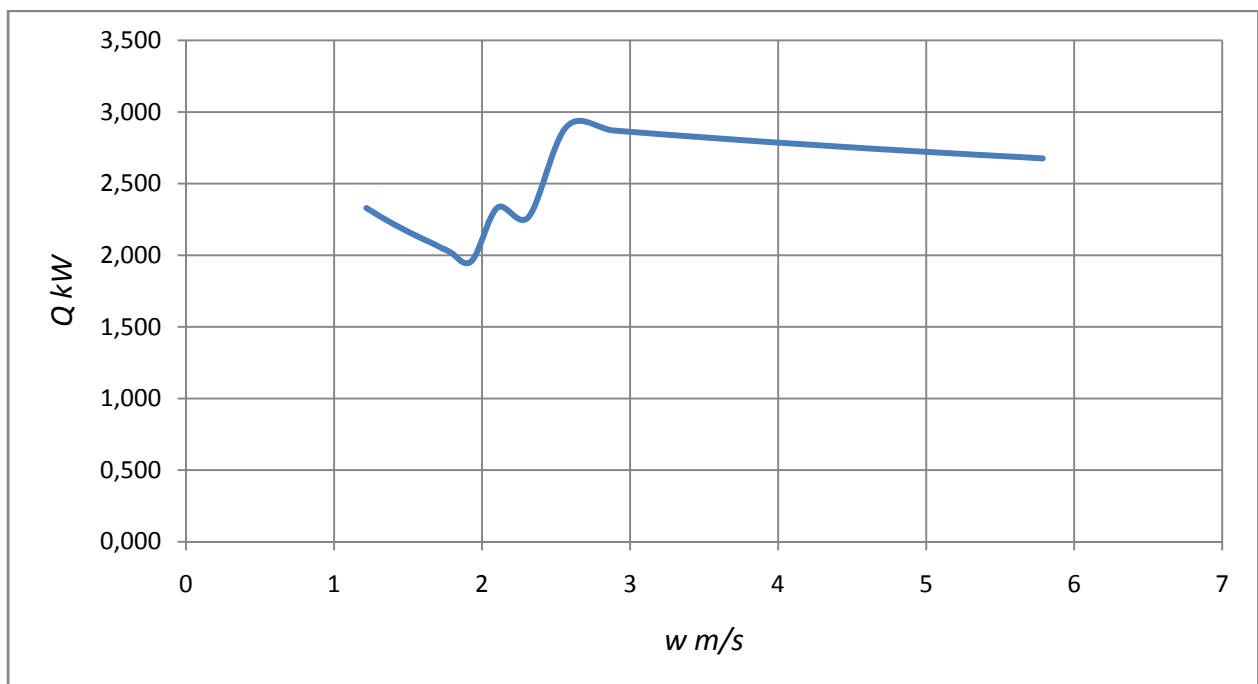
Slika 27. Ovisnost toplinskog toka Q o brzini strujanja uz protoke zraka q_v = 500 \text{ m}^3/\text{h} i pri vanjskoj temperaturi \theta_1' = -15 °C
