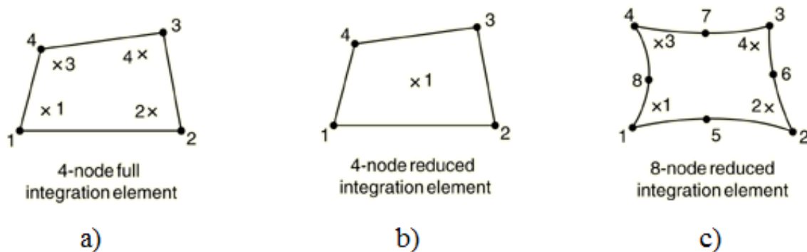
Slika 2.2. Točke integracije za element: a) S4, b) S4R, c) S8R [4]
