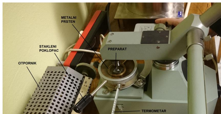
Slika 5.13. Polarizacijski mikroskop za određivanje tališta
