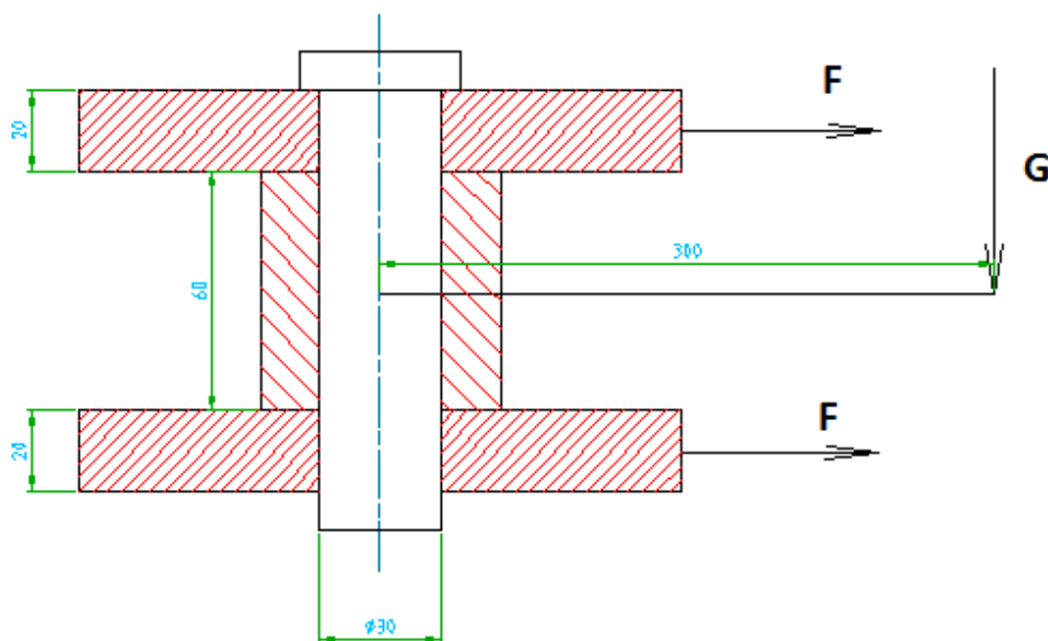
Slika 22. Presjek svornjaka
