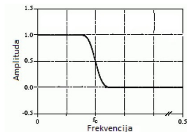
Slika 6.7. Rezultat impulsnog odziva filtera
