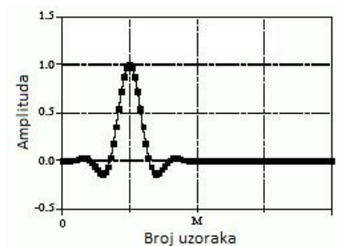
Slika 6.6. Rezultat množenja Blackamanovog vremenskog prozora sa funkcijom sinc
